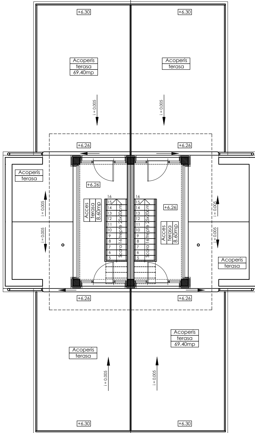
Acces Terasa_Poz.4 ÷15. Ap: C25-A ÷ C36-A 4 CAMERE
