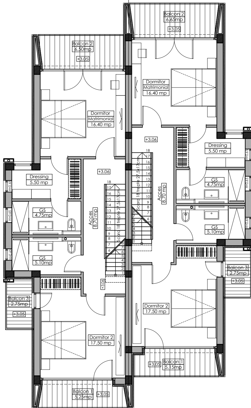
Etaj 1_Poz.1. Ap: C22-B 4 CAMERE
